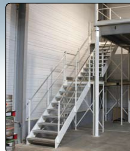
Escalier avec palier Plancher à 4 m et plus.
